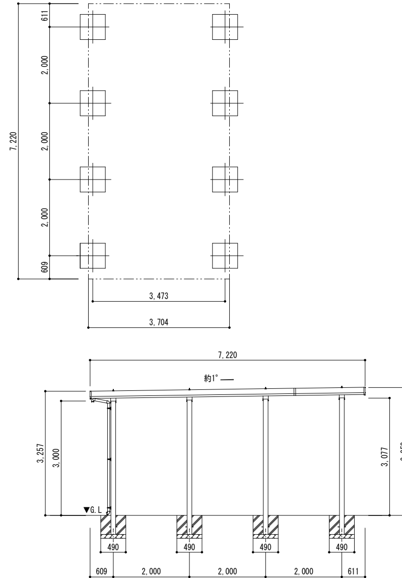
■ 基礎配置図
