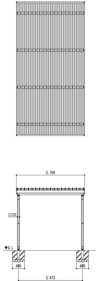
■ 接図
